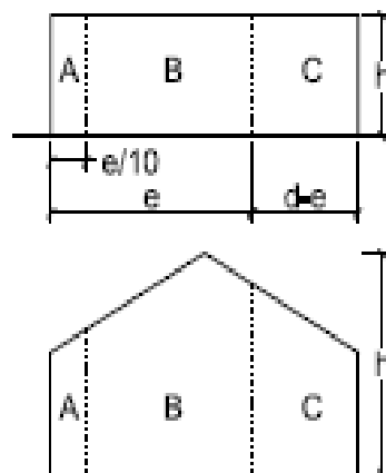
Ejemplos de alzados
